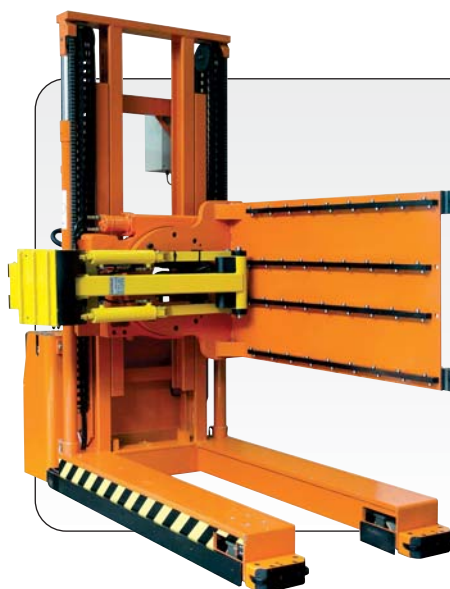
Double système tire pousse : traverse motorisée + vérins télescopiques
