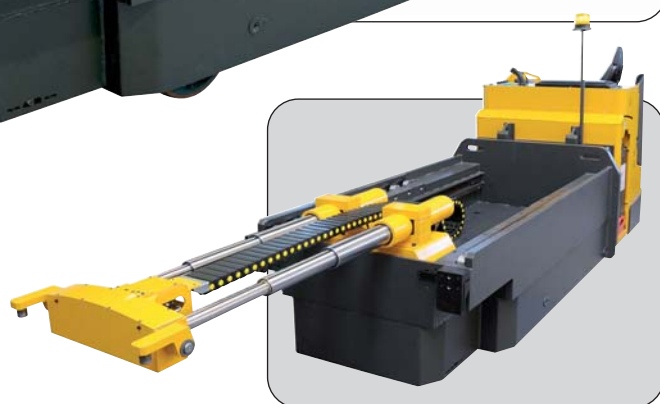
Double système tire pousse : traverse motorisée + vérins télescopiques
