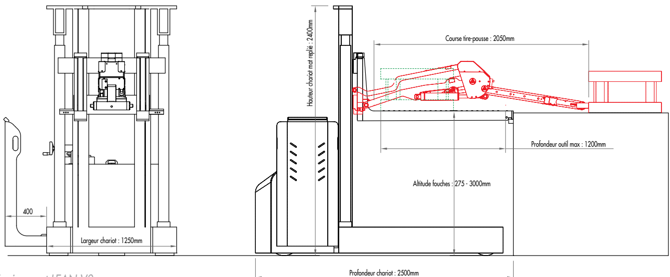
Rack de stockage outil CANTIBLOC®, 5 niveaux de stockage, altitude du dernier niveau : 2900 mm
